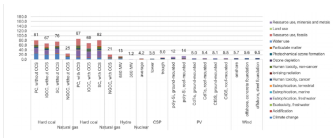
Figura 1. impactos ambientales normalizados del ciclo de vida, ponderados por 1 TWh de producción, por tecnología Europa, 2020
